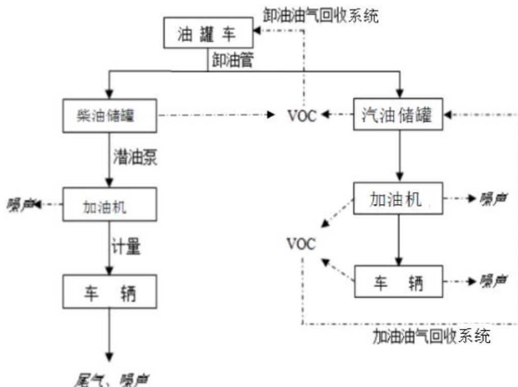
图 2-2 运营期生产工艺与产污节点图
