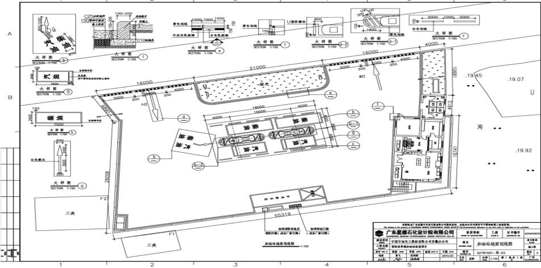
附图 3 中国石化销售有限公司安徽安庆石油分公司凉亭河加油站建设项目平面布置图
