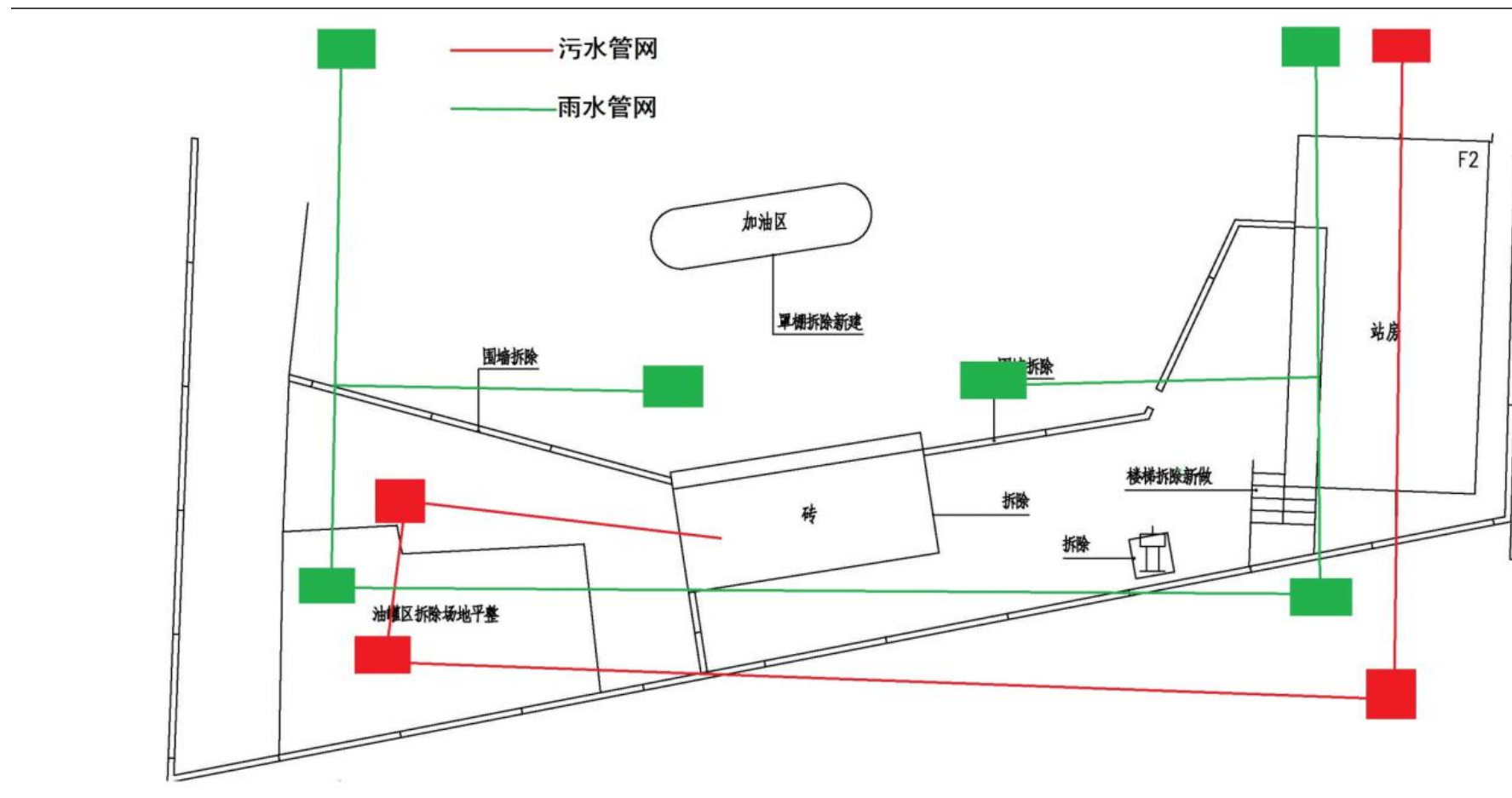
附图 4 中国石化销售有限公司安徽安庆石油分公司凉亭河加油站建设项目雨污分流图
